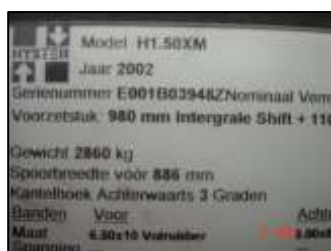
Plaque constructeur
